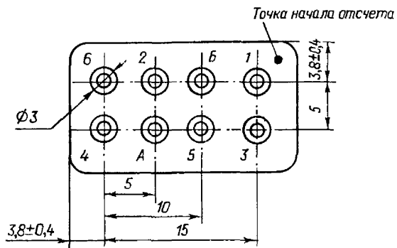
Рис. 2-35. Конструктивные данные и маркировка выводов реле РЭС47
